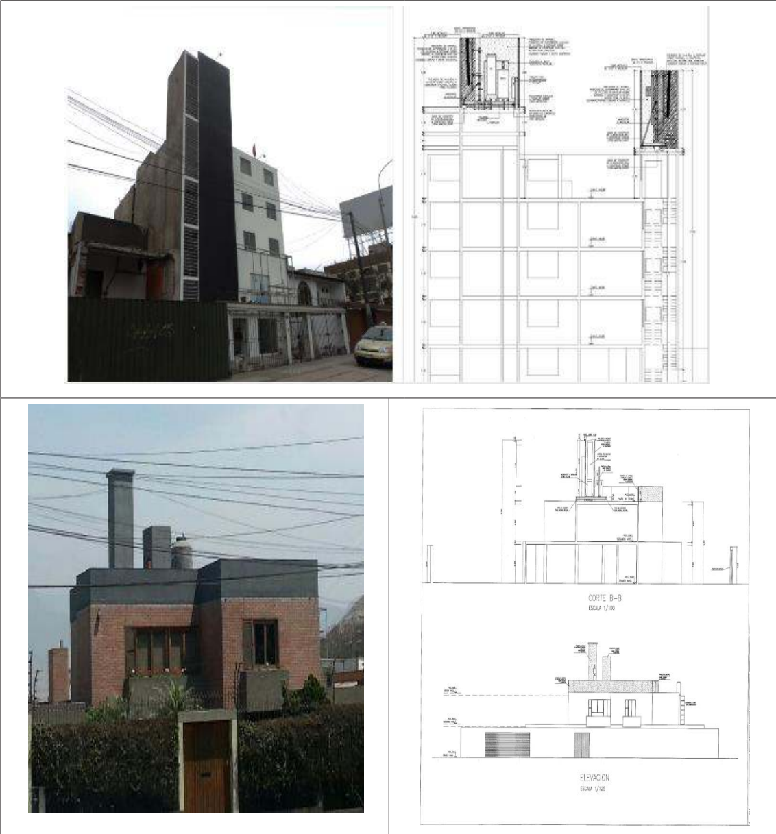
Figura N° 12: Mimetizado tipo Paneles de Lamas
