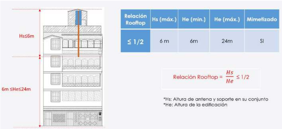
Figura N° 9: Relación de alturas para mimetizados tipo Rooftop
