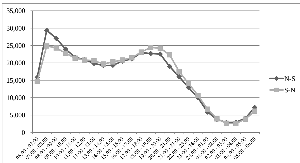
Figura 2.13 Volumen de Tránsito por Hora en la Línea Cortina del río Rímac (Vehículos/día)
