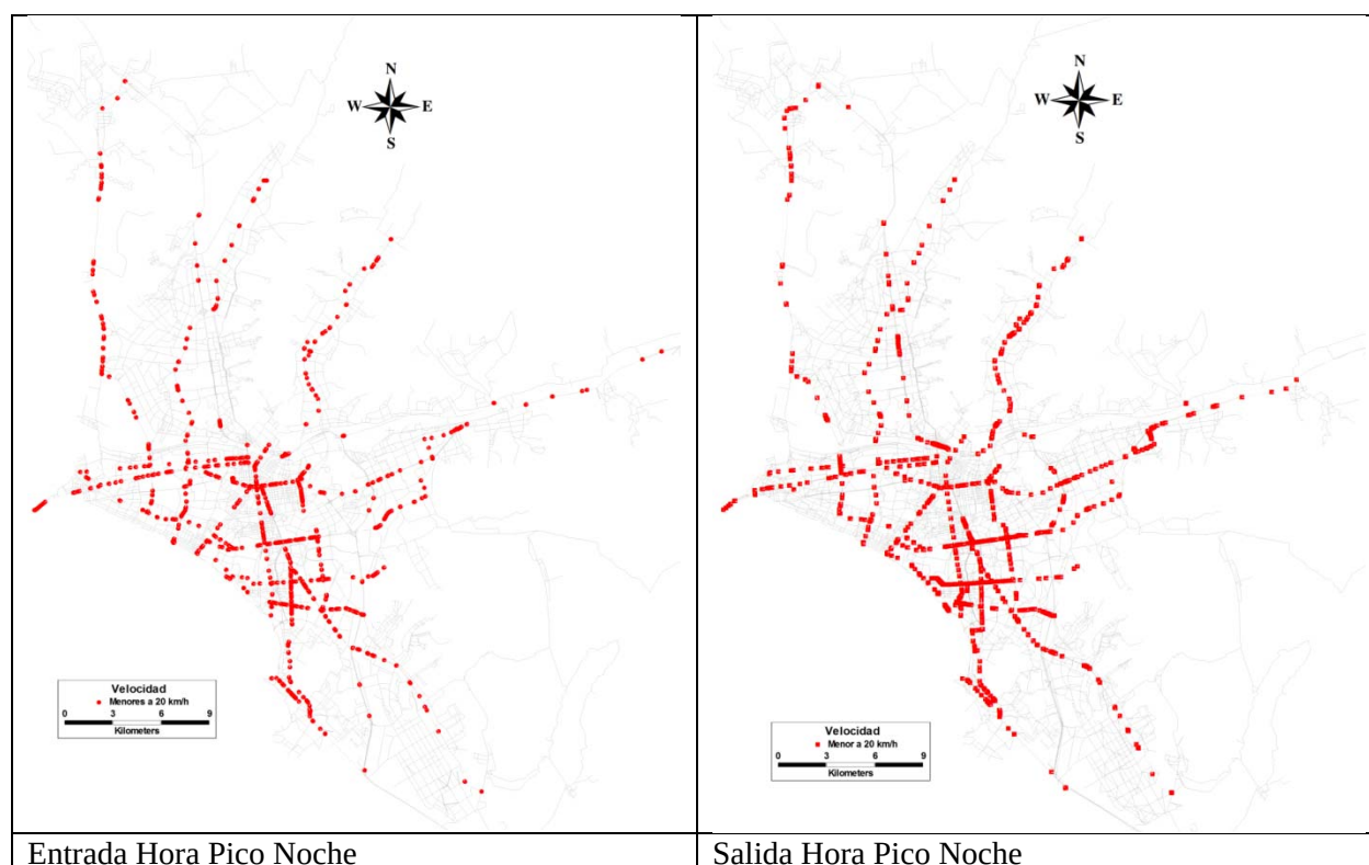
Figura 2.17 Vías principales con Velocidades de Viaje Menores a los 20km/h
