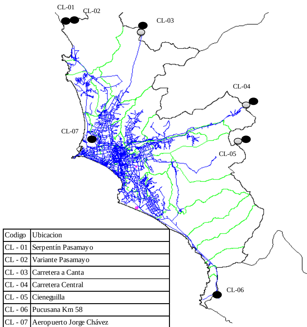
Figura 2.7 Ubicación de los puntos de conteo de la Línea Cordon
