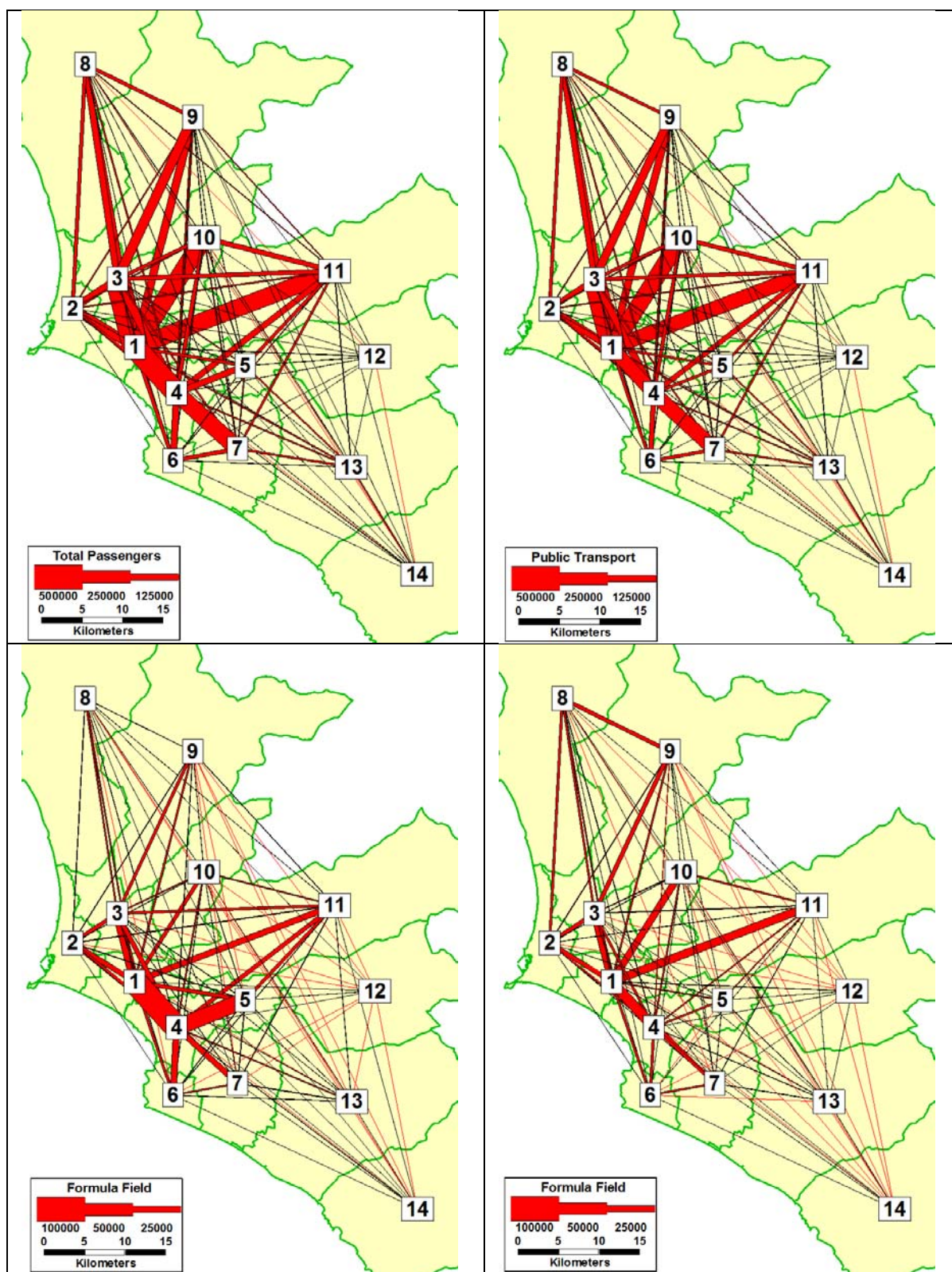
Figura 3.20 Líneas de Deseos de Viajes
