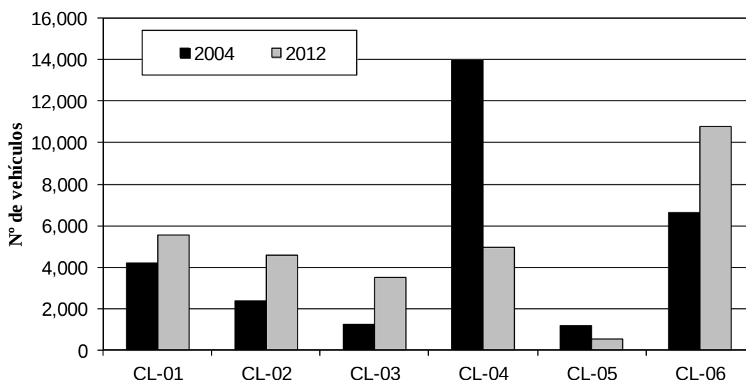
Figura 2.8 Comparación del Volumen de Tráfico en la Línea Cordón
