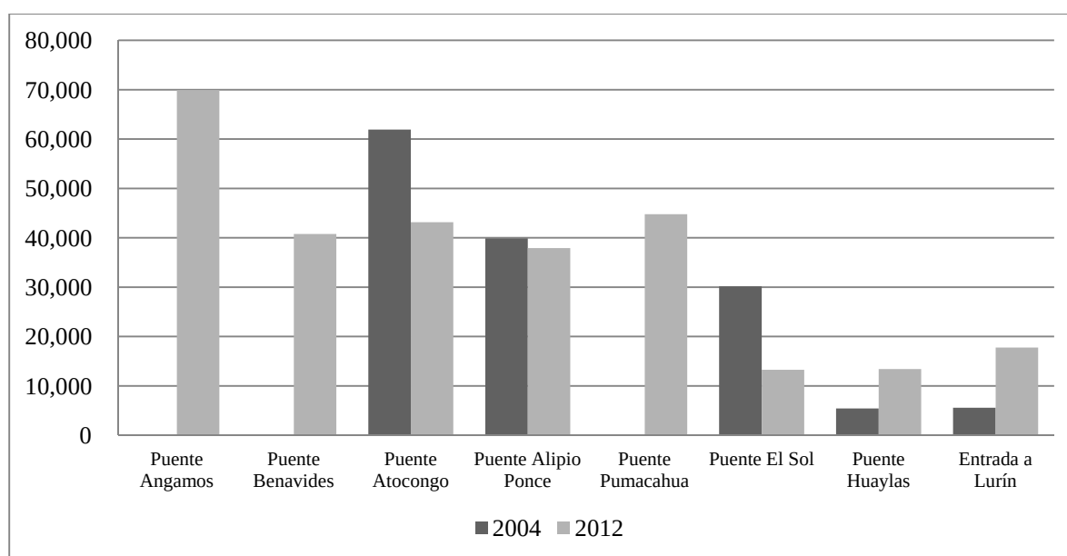
Figura 2.12 Volumen de Tráfico que cruza la Línea Cortina de la Panamericana Sur
